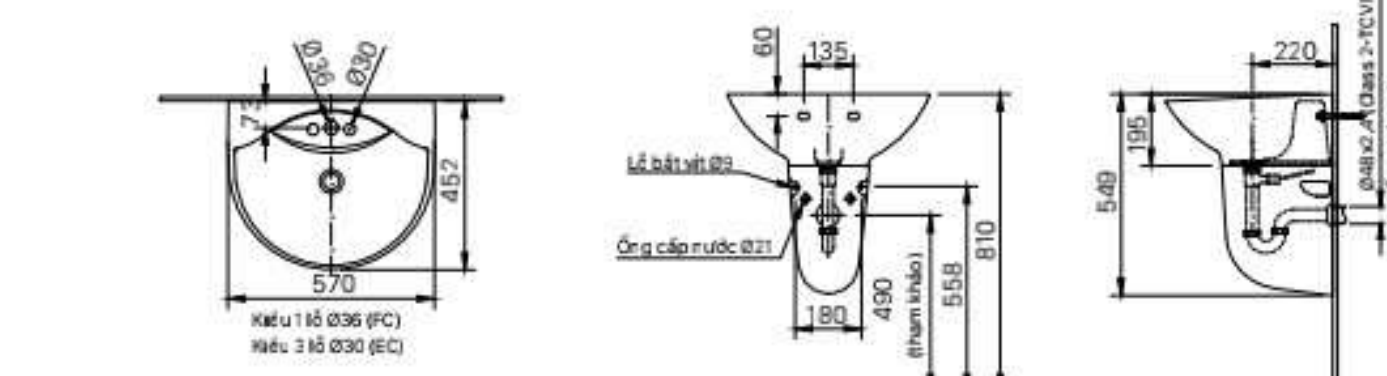
L-288V (EC/FC) | L-288VC (CHÂN CHẬU)
