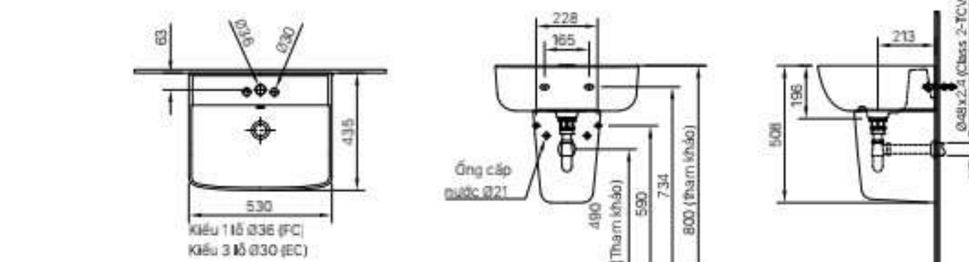
AL-312V | L-312V | L-298VC(chân chậu)
