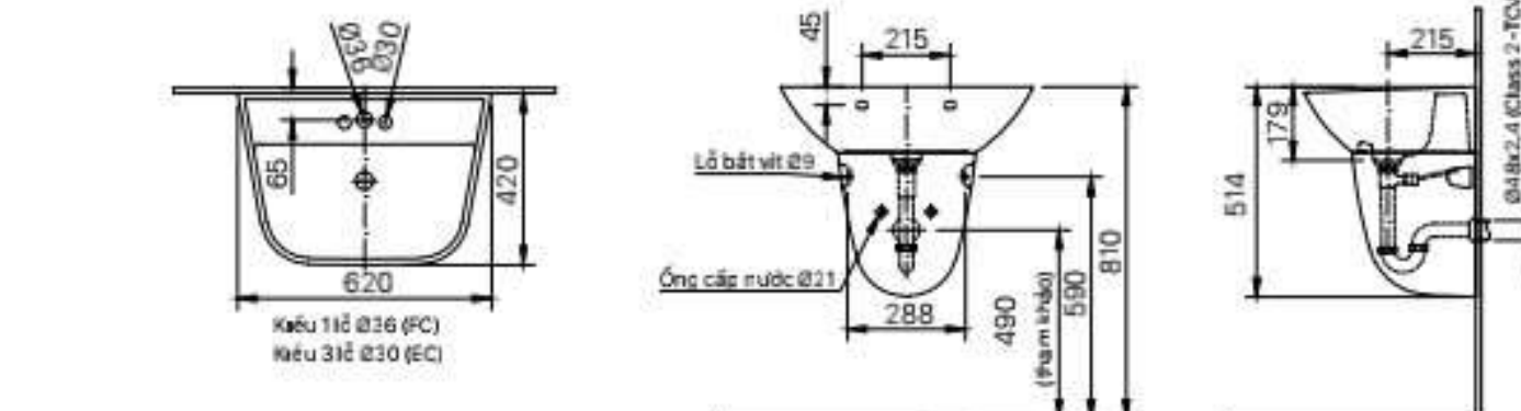
L-297V (EC/FC) | L-297VC (CHÂN CHẬU)
